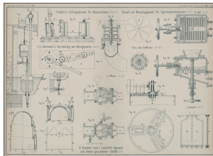
Szkice do patentu Woesslera.
